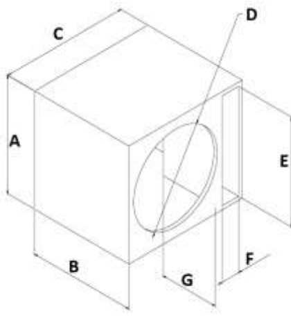
CAIXA DUTO RETANGULAR / RECTANGULAR DUCT BOX
